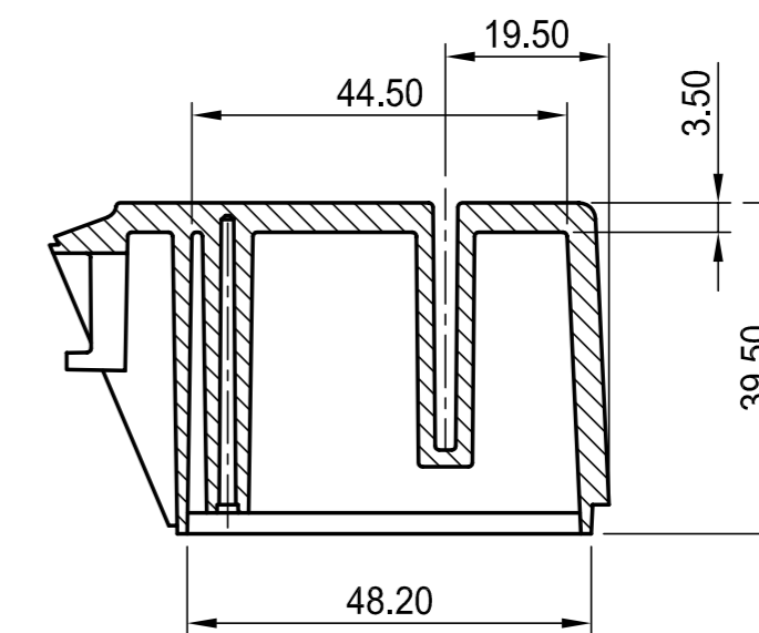
SCHNITT A-A section
