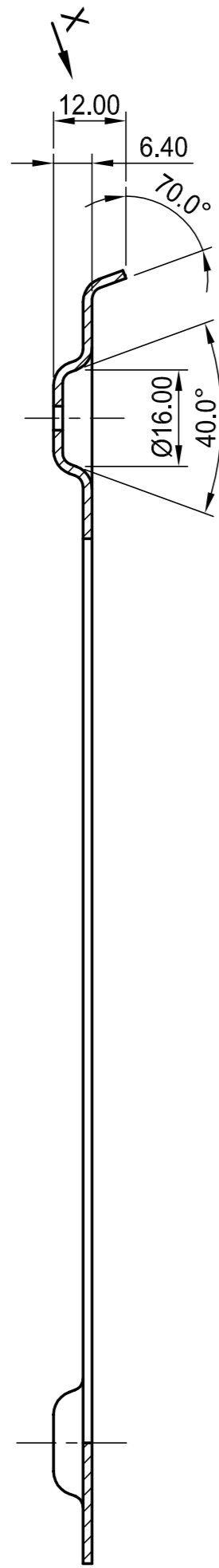
SCHNITT A-A section
